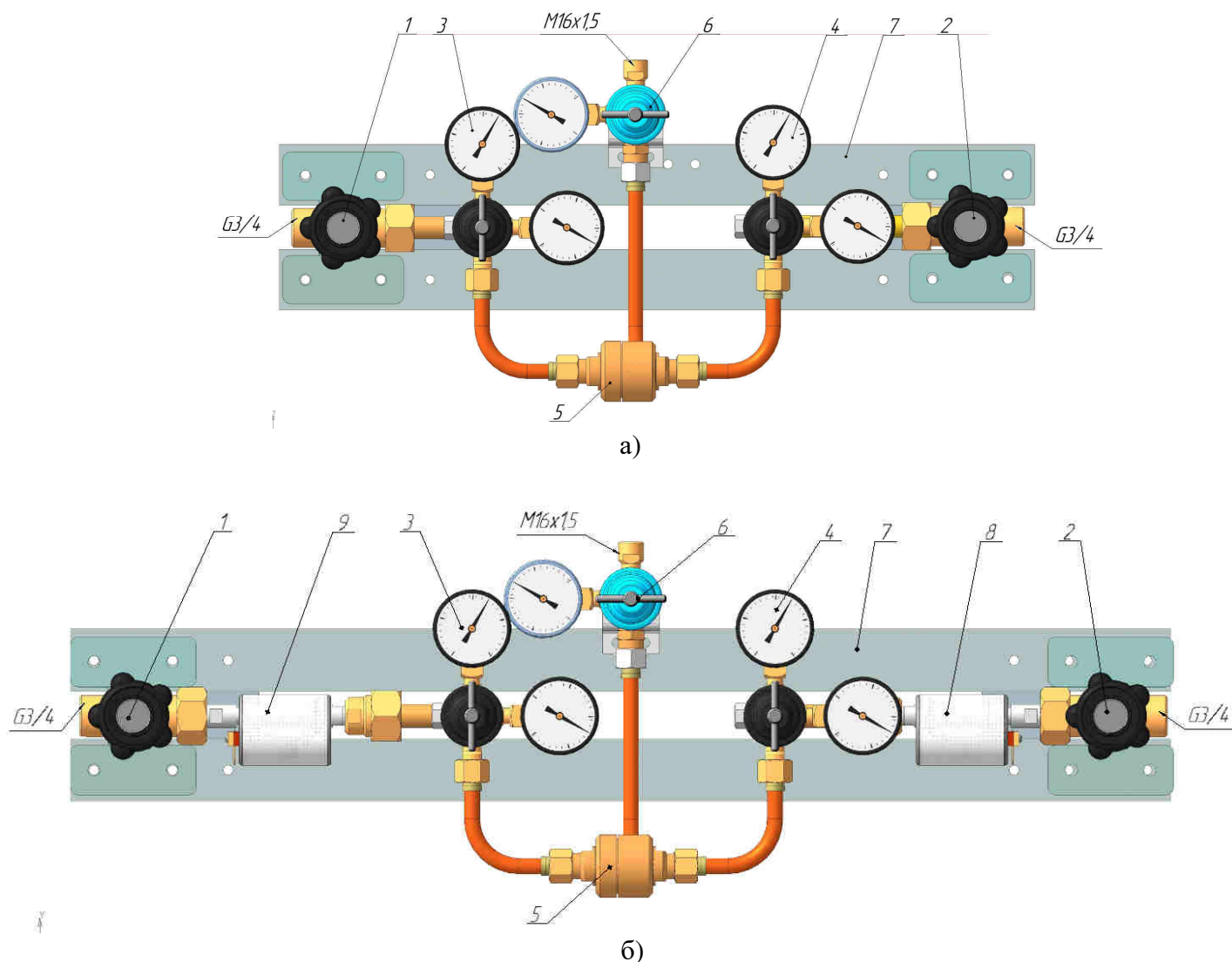
Рис.1 Щит автопереключения плеч перепускных газовых рамп.
